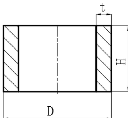
图1 筒形锻件有效厚度示意图
