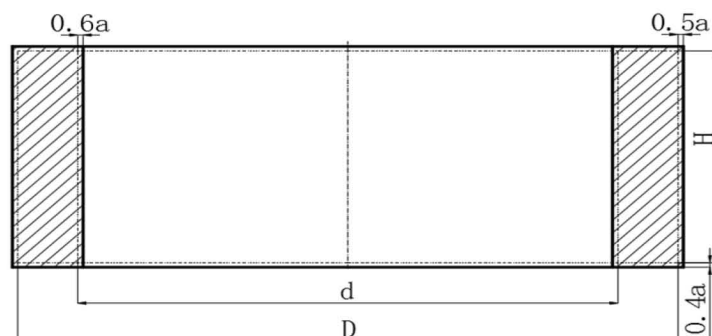
图2 筒形锻件轮廓图
