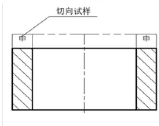
图3 筒形锻件取样位置
